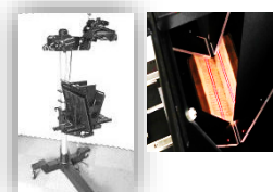
開発品 : 貴重洋書用 30度見開きデジタル撮影システム
